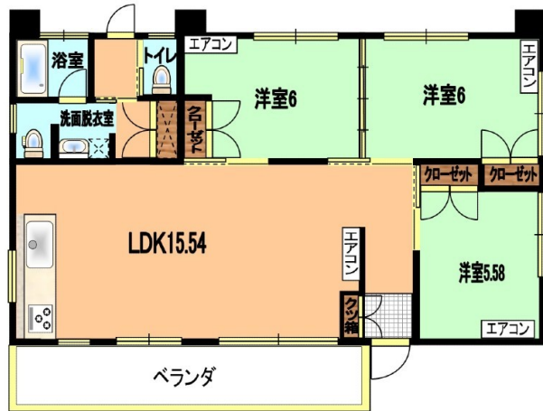
物件間取
