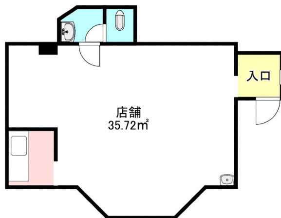
物件間取
